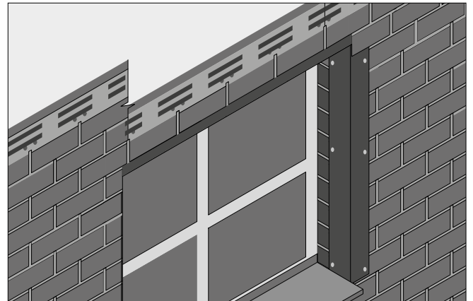
Рис. 18. Монтаж фасадной плитки поверх оконного наличника сверху проема
