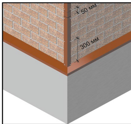
Рис. 16 Устройство внешних углов при помощи металлических уголков.
